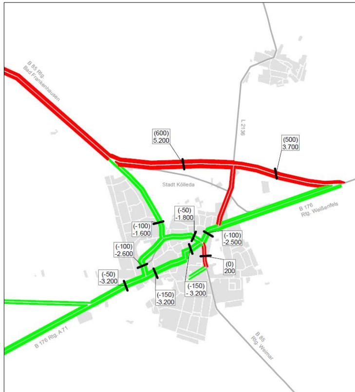
Abb. 7: Differenzenplan – Planfall– Ortsumfahrung / Analysefall [Kfz/24 h]
